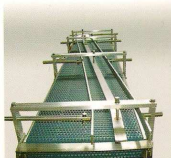
Trasporto motorizzato per vaschette plastica Powered conveyor for plastic jars
