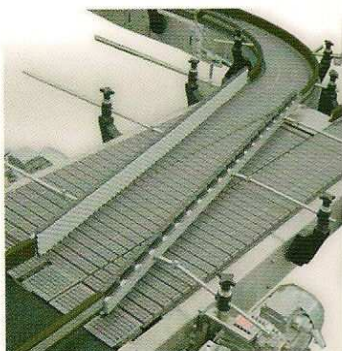
Trasporto fardelli con deviazione da due linee ad una linea Pack conveyor with change from two line to one line
